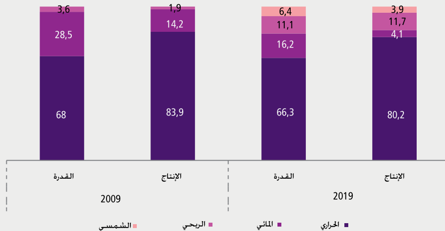
رسم بياني 2.1.2.1: هياكل القدرة المنشأة وإنتاج الكهرباء حسب المصدر (%)
