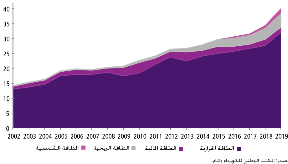
رسم بياني 4.2.1: إنتاج الكهرباء حسب المصدر (بآلاف جيجاواط ساعة)
